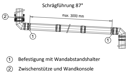
Bilder: Schrägführung
